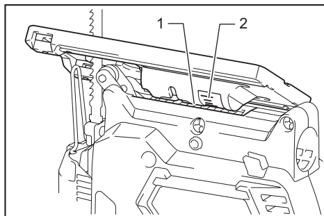
► 1. Borde 2. Graduación
